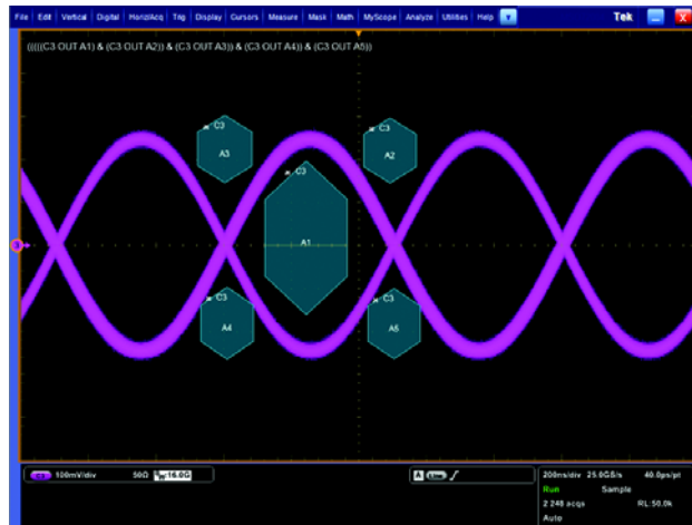
使用选项可视触发的触发眼图
